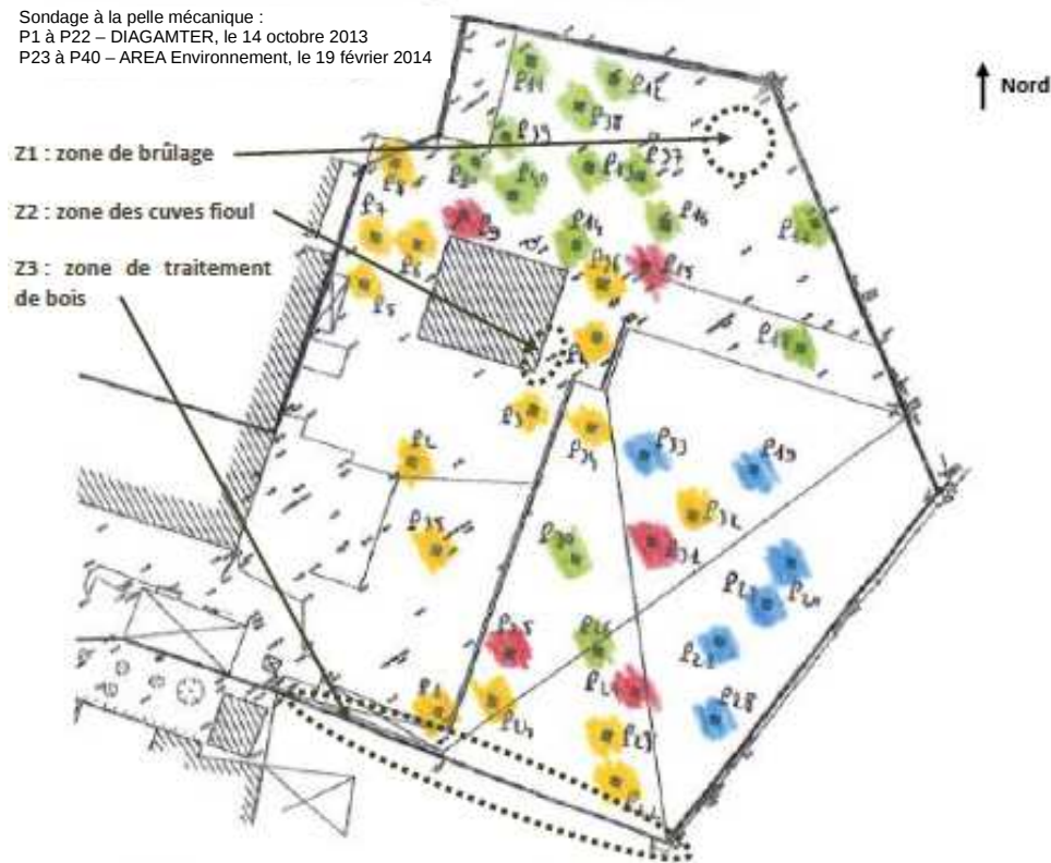
2 - Carte de présence de fragments de fibrociment au droit des sondages de reconnaissance
