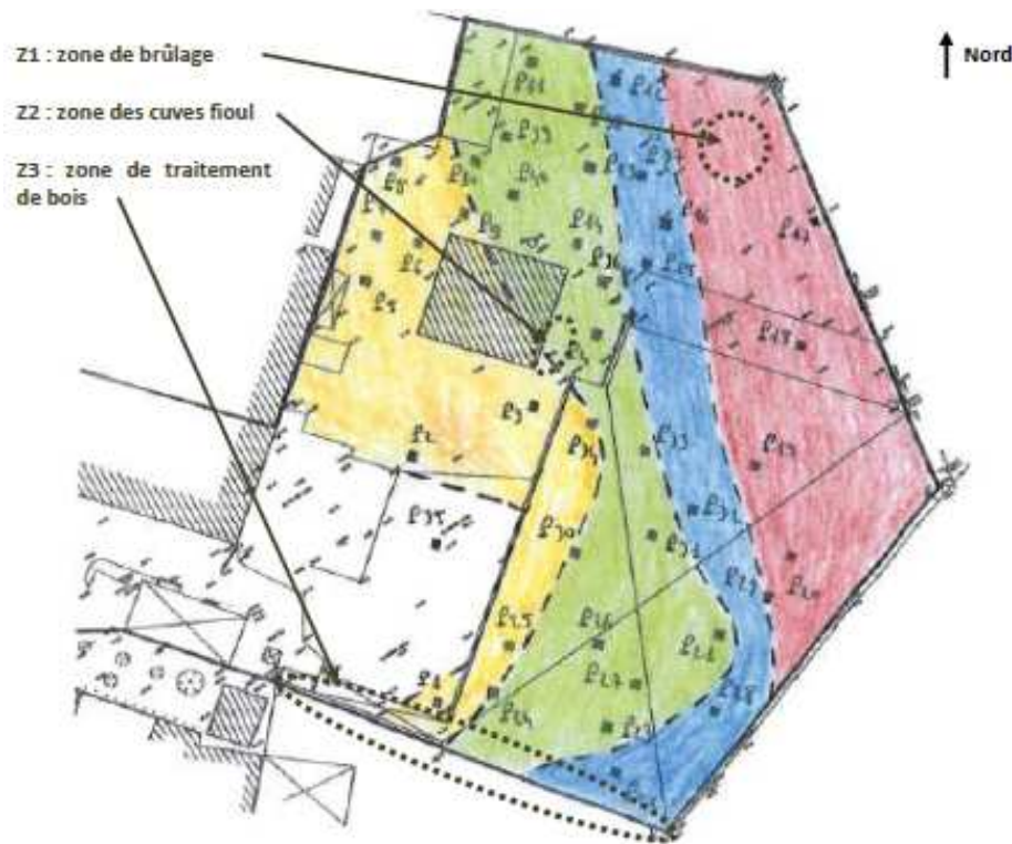
1- Plan d'implantation des sondages de reconnaissance avec épaisseur des remblais présents sur site
